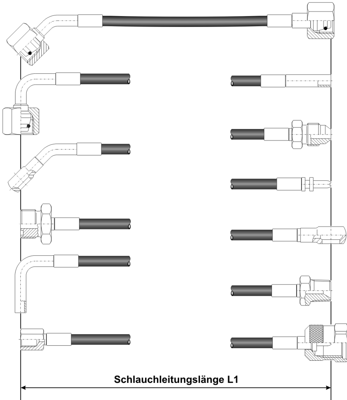
Abbildung 1: Schlauchleitungslängen
